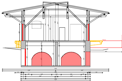
Carl-Thieme-Str. Schnitt AA Halle
